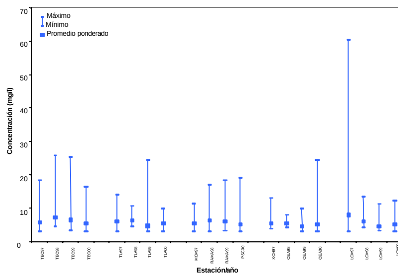
Gráfica 3.20 \text{SO}_4^{=} en depósito húmedo 1997-2000.
