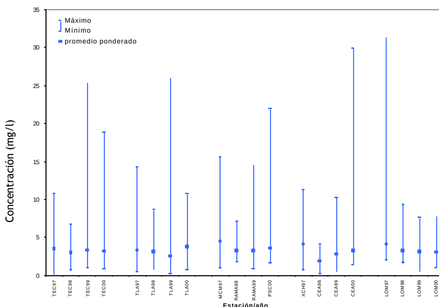
Gráfica 3.19 \text{NO}_3^- en depósito húmedo 1997-2000.
