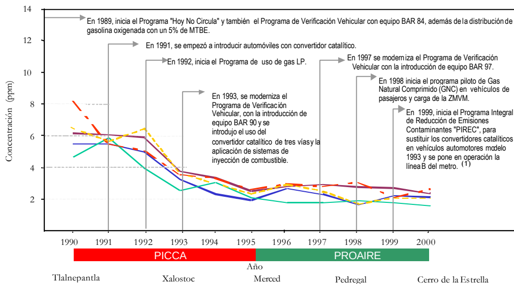
Gráfica 1.3 Tendencia del monitoreo atmosférico de monóxido de carbono y principales acciones para reducir sus emisiones en la ZMVM, 1990-2000.
