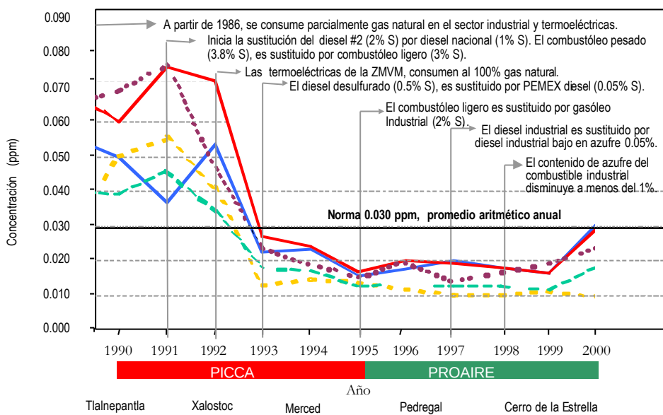
Gráfica 1.2 Tendencia del monitoreo atmosférico de bióxido de azufre y principales acciones para reducir sus emisiones en la ZMVM, 1990-2000.
