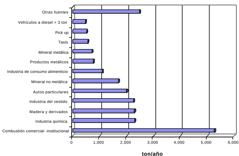
Gráfica 5.4 Contribución de SO_2 por fuentes.
